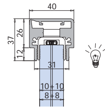
B-3020 Corrimano quadro. Square handrail profile. Quadrat Handlauf Profil.
