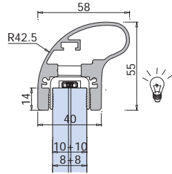
B-3010 Corrimano tondo. Round handrail profile. Rund Handlauf Profil.
